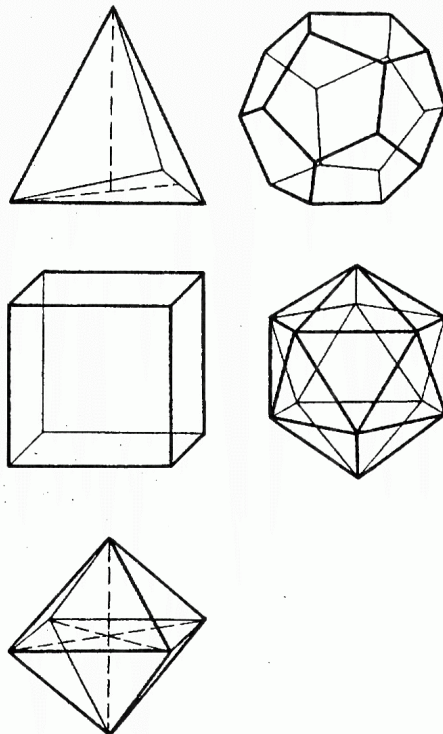
Die fünf platonischen Weltkörper: Tetraeder, Würfel, Oktaeder, Pentagondodekaeder und Ikosaeder.
