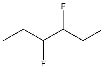
3,4-difluoro-hexane
